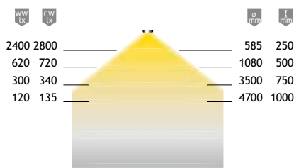
Lichtverdelingsdiagram 120°
