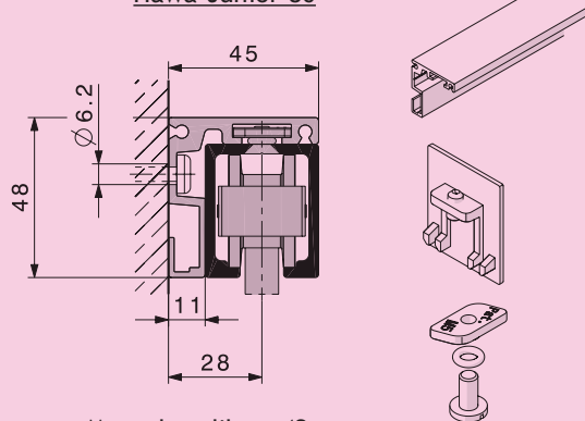
Hawa-Junior 80
