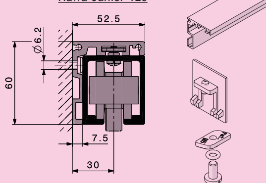
Hawa-Junior 120
