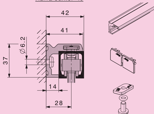
Hawa-Junior 40
