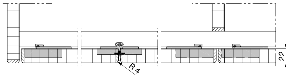
portes intégrées au corps
