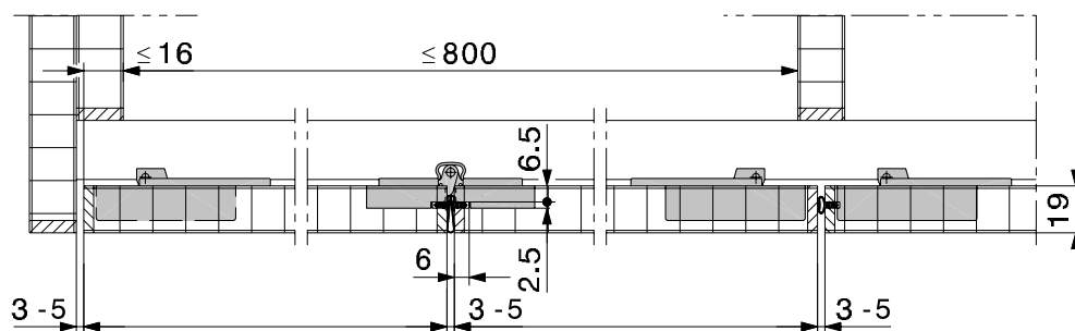
portes semi-intégrées au corps avec panneau latéral apparent
