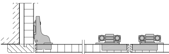
portes coulissant devant le corps
