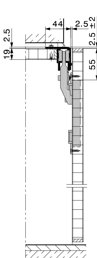
portes coulissant devant le corps
